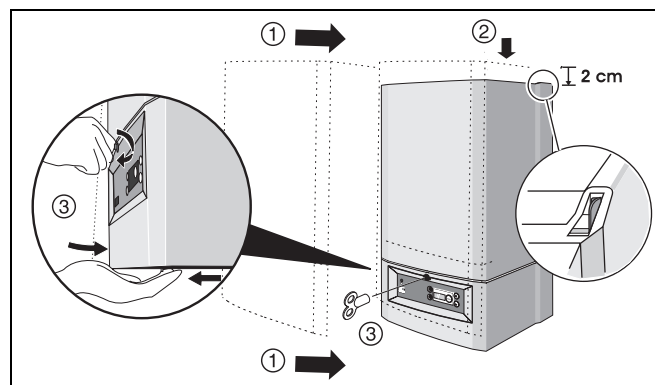
Рис. 37 Установка кожуха
