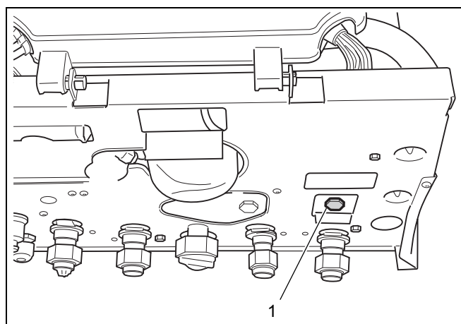
Рис. 7 Позиция заглушки
