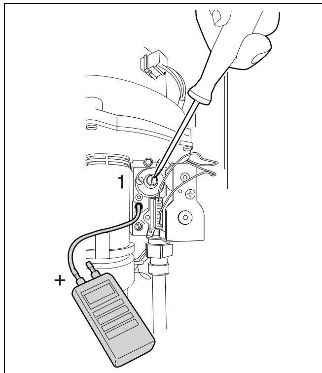
Рис. 34 Установка соотношения газ/воздух
