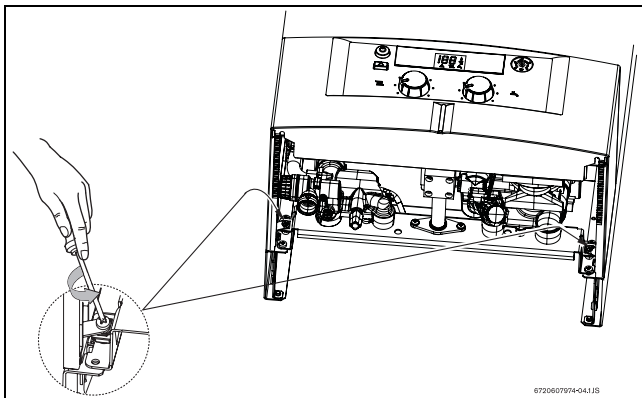
Рис 9 Расположение винтов
