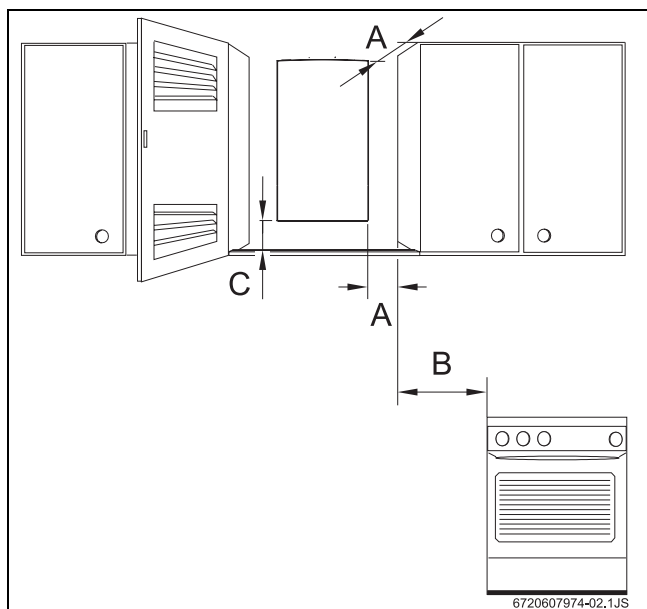
Рис 7 Минимальные расстояния
