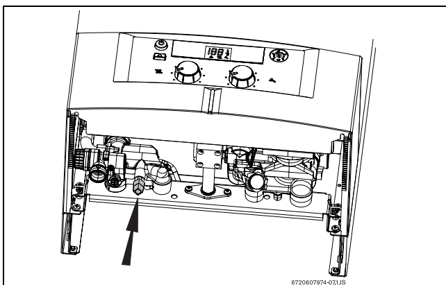
Рис 16 Кран подпитки
