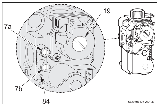
Рис 27 Газовая арматура
