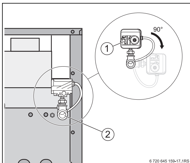
Рис. 9 Подключение газа
