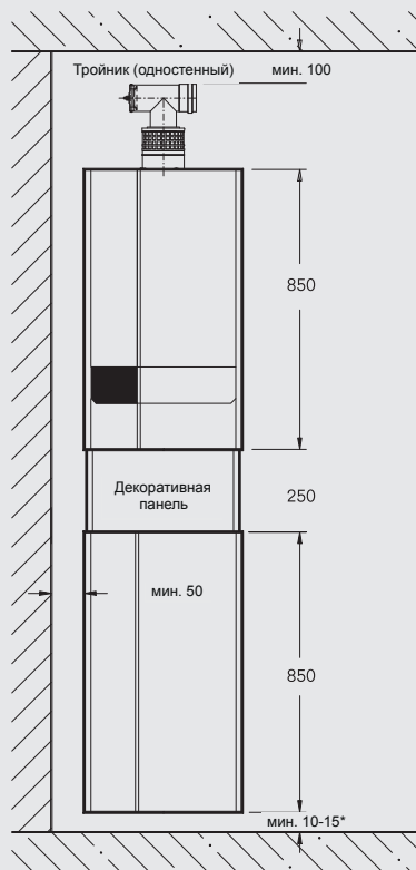
Монтаж под циркуляционным водонагревателем
