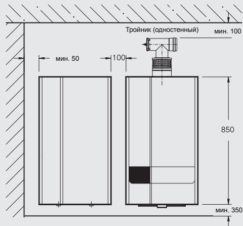
Монтаж рядом с циркуляционным водонагревателем
