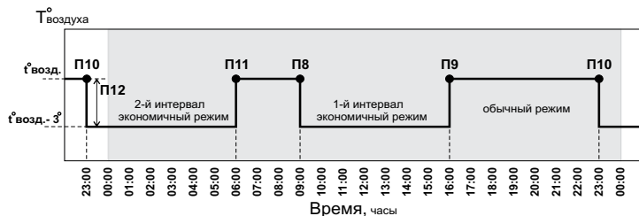
Рис.4 График температуры воздуха в помещении для Режим 1.
