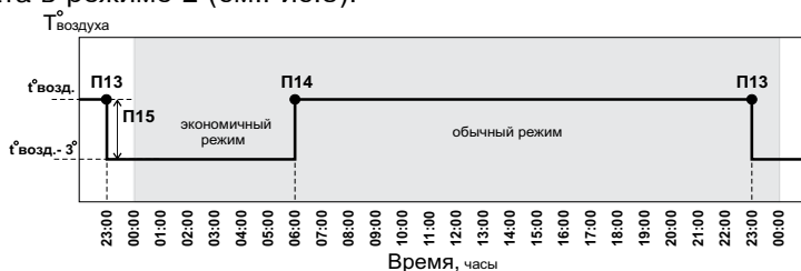
Рис.5 График температуры воздуха в помещении для Режим 2.
