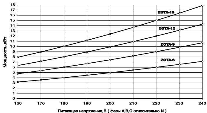
Рис.8 График изменения мощности водонагревателя в зависимости от питающего напряжения
