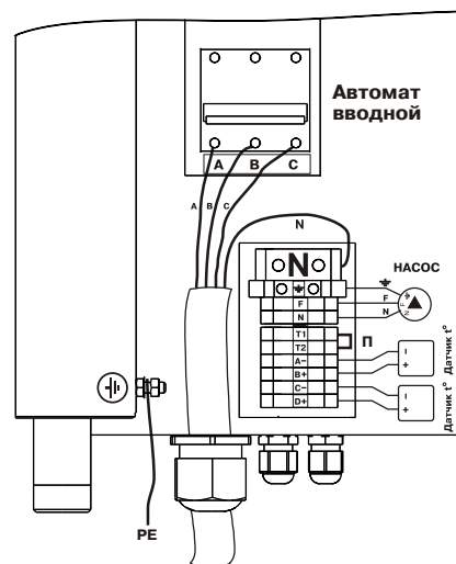
Рис.3 Схема подключения водонагревателя к сети переменного тока
